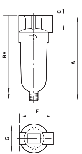
Автоматический дренаж
