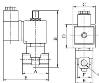
Габаритные размеры (мм)
